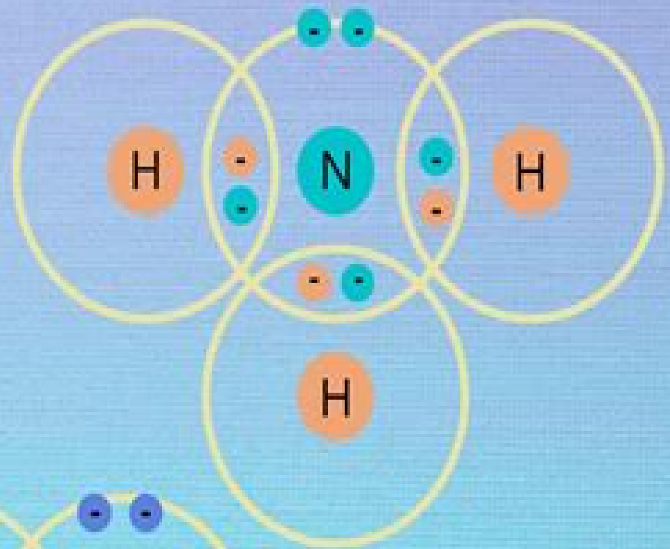
Ammonia (NH 3 )
