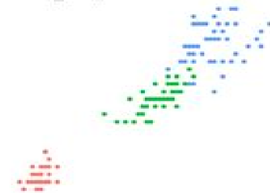
theme_void()
