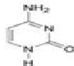
cytosine
