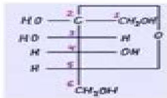
β-D (-) fructofuranose
