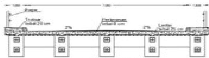
PENAMPANG UJUNG
