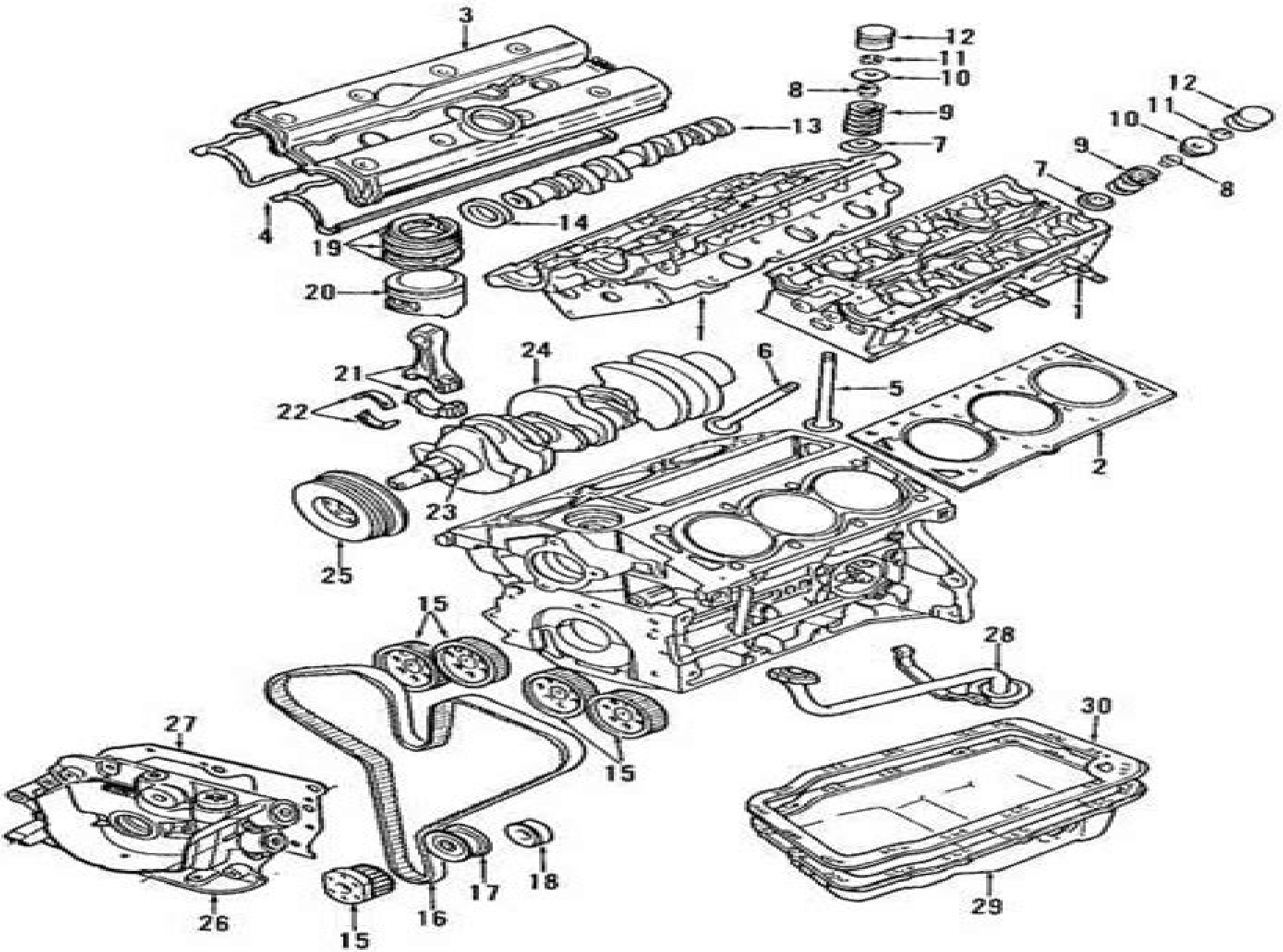
ENGINE-2.5L D.O.H.C.
