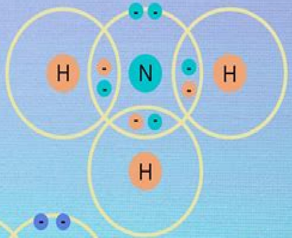
Ammonia (NH 3 )
