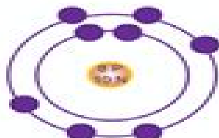
^{18}\text{O} Isotope
