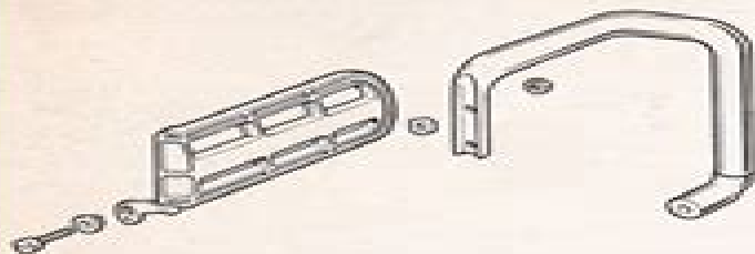
MONTAGGIO PARAMANO MONTAGE DU PROTEGE-MAIN HAND GUARD ASSEMBLY MONTAJE DEL MANSCHUTZES MONTAJE DE PROTECCION
