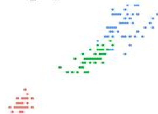
theme_void()
