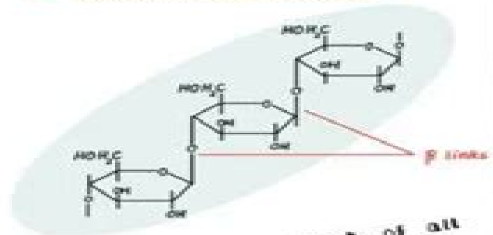
β-D (-) fructofuranose
