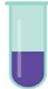
LITMUS
