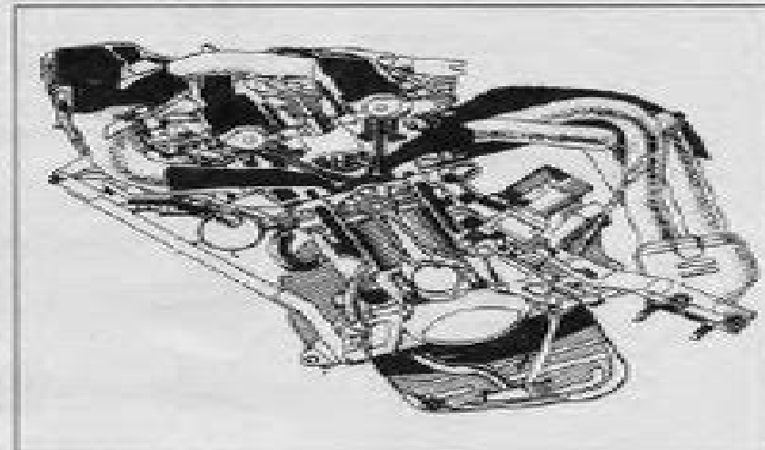
Двигатель 3S-GE.
