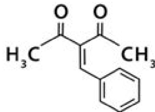
3-Benzylidene-2,4-pentanedione
