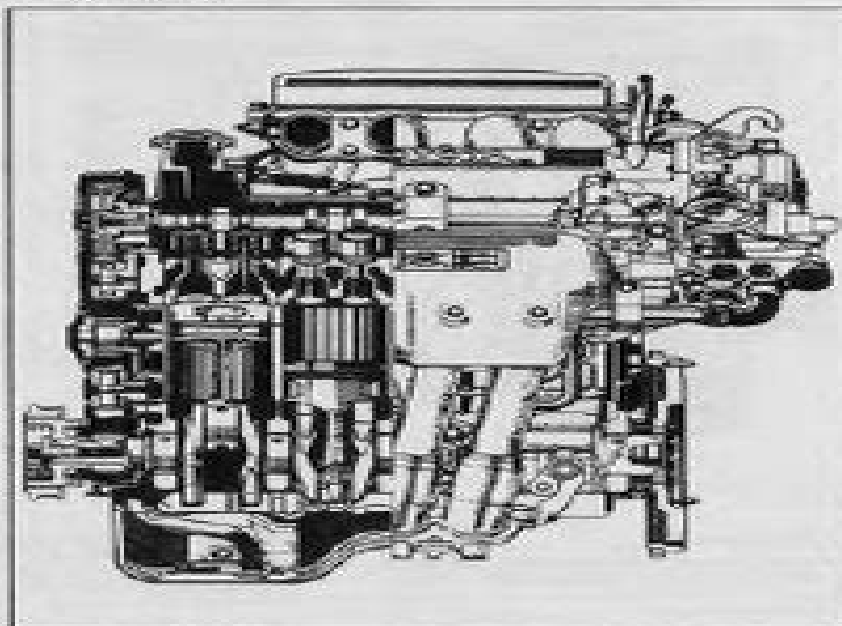
Двигатель 3S-GE.
