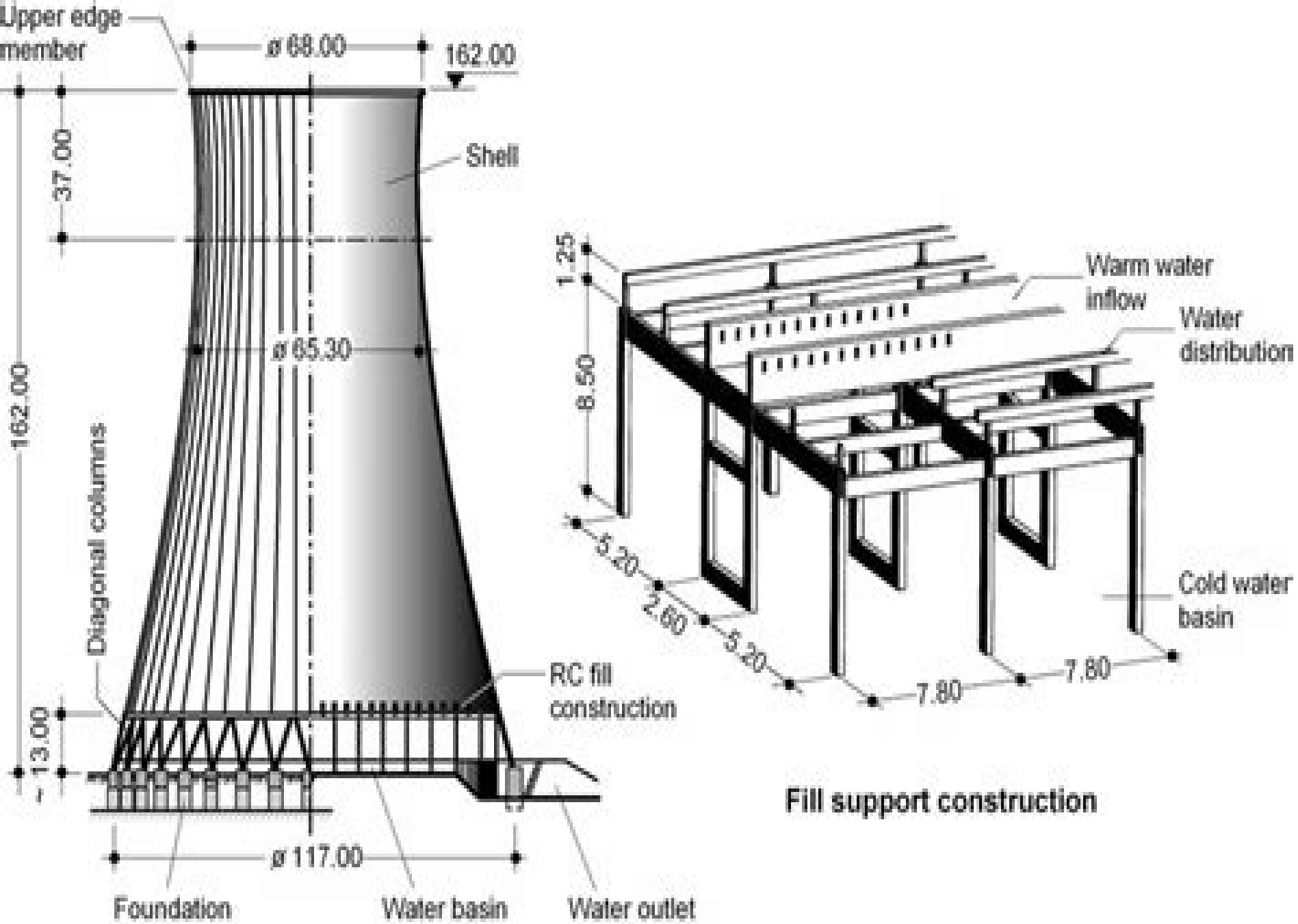
Natural draft cooling tower (Mülheim-Kärlich)
