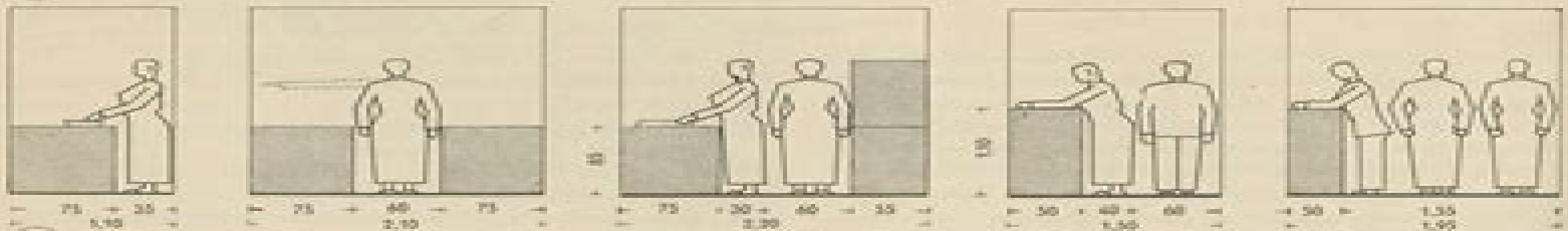
4 Platzbedarf zwischen Möbeln
