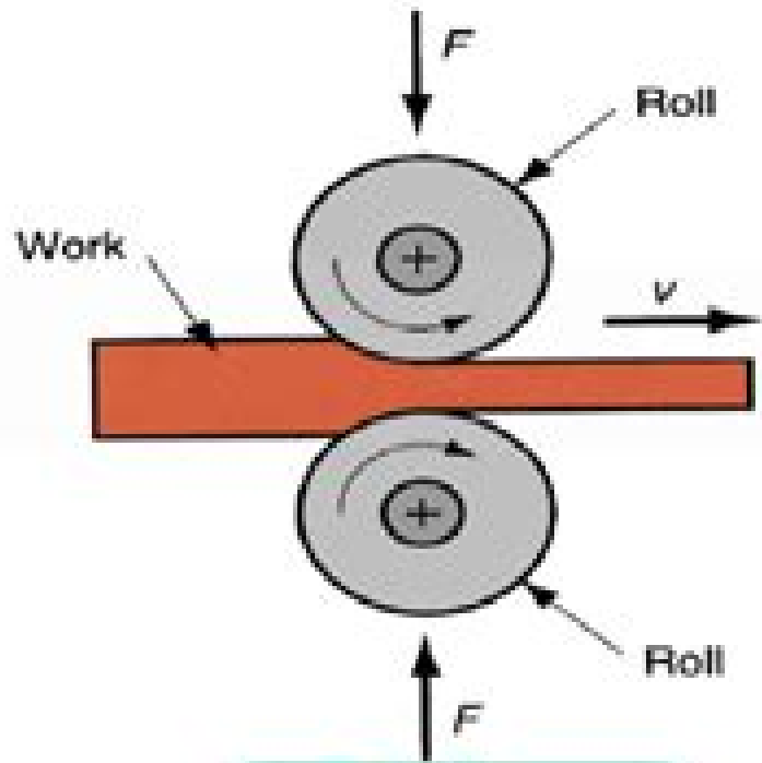
Rolling
