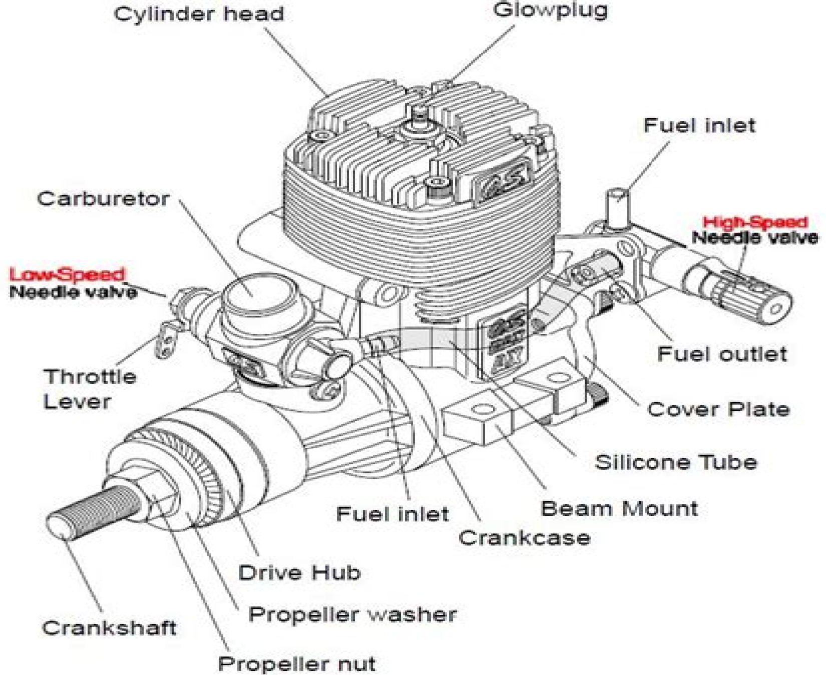
O.S. 46AX
