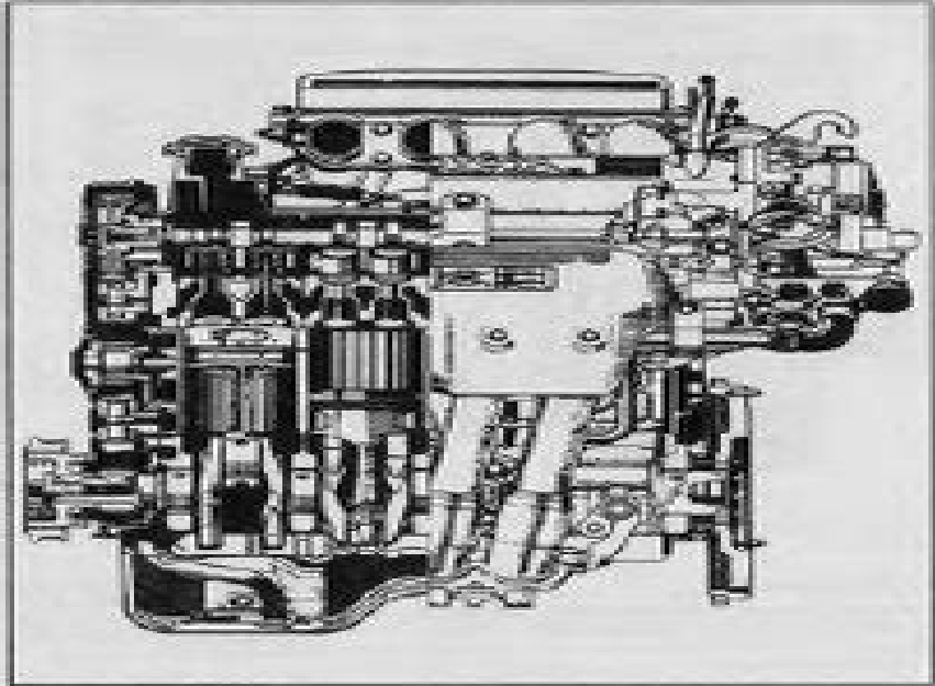
Двигатель 3S-GE.
