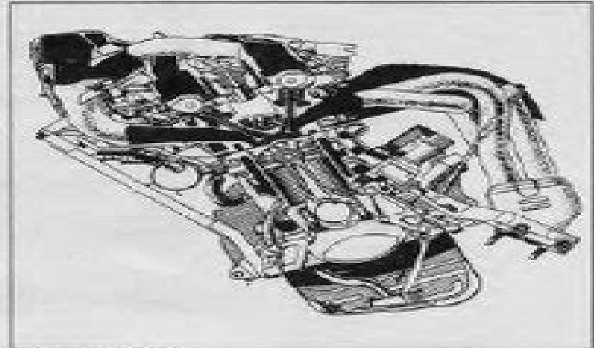
Двигатель 5S-FE.
