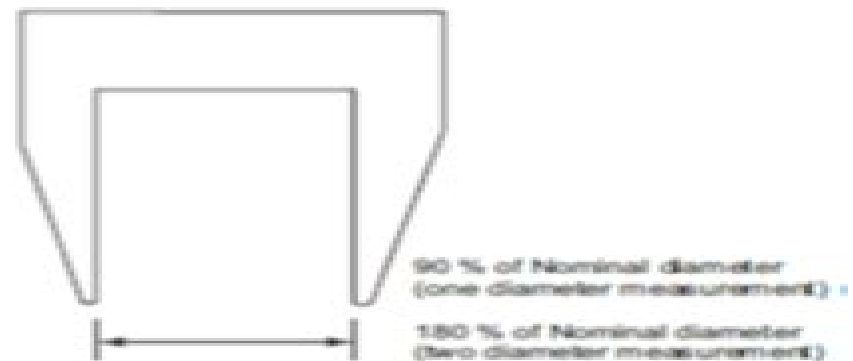
e) Go-no-go gauge
